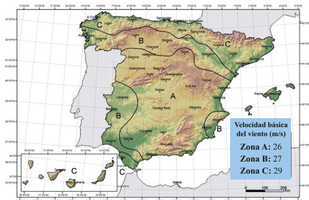
Figura 1 - Valor básico de la velocidad del viento, vb
